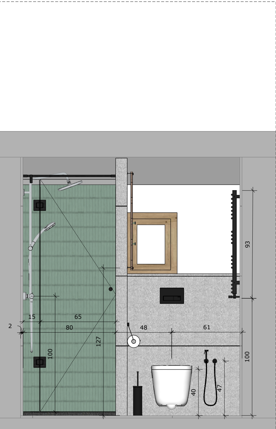
PRZEKRÓJ F-F _SKALA 1:20
