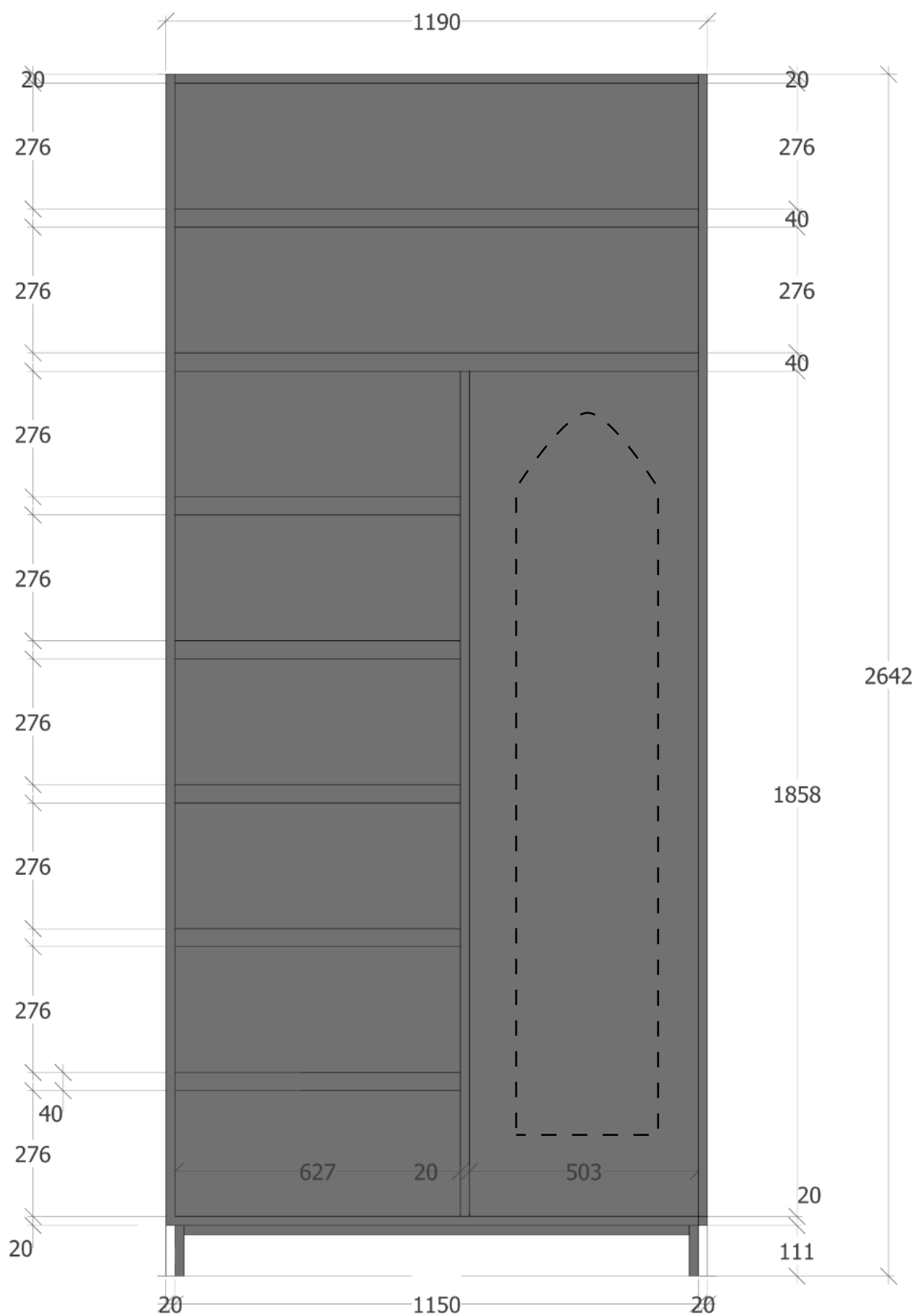
WIDOK FRONTU (BEZ WIDOCZNYCH FRONTÓW)
