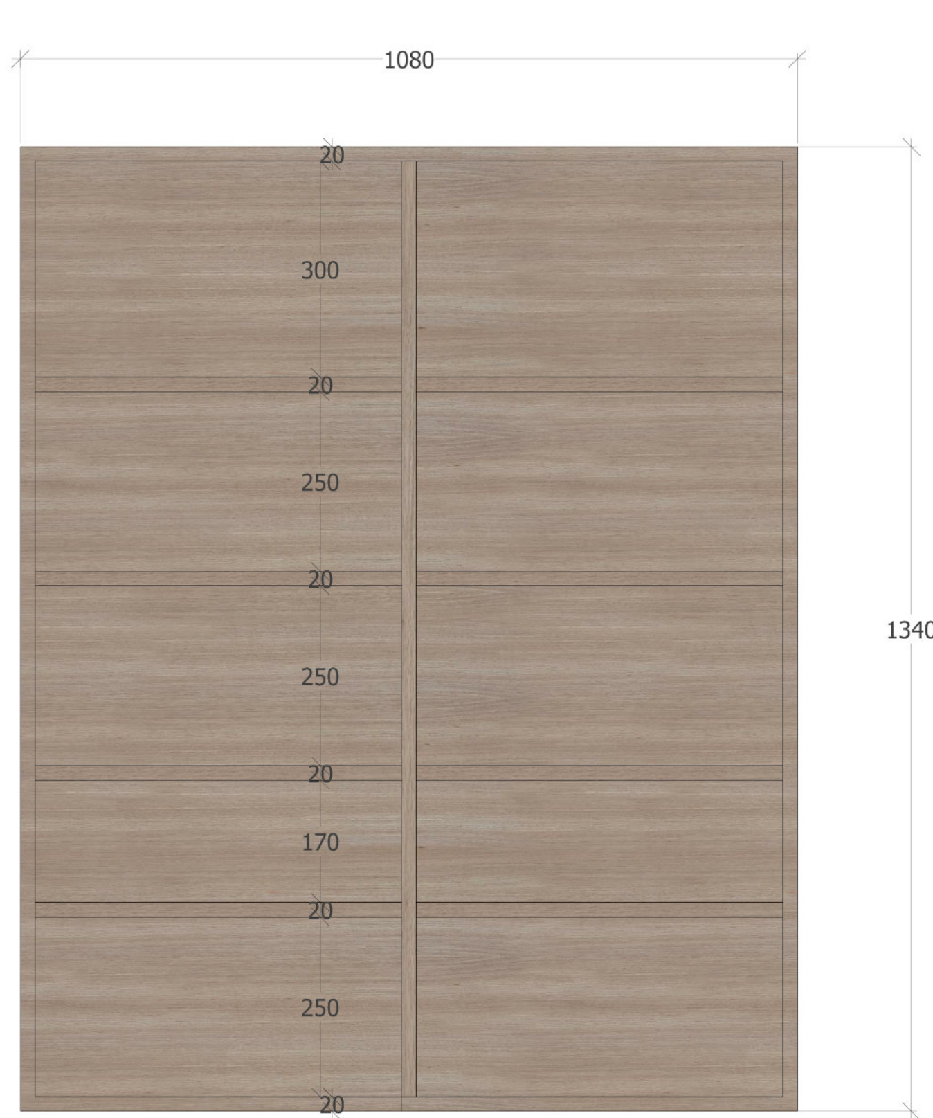
WIDOK OD FRONTU (BEZ WIDOCZNYCH FRONTÓW)
