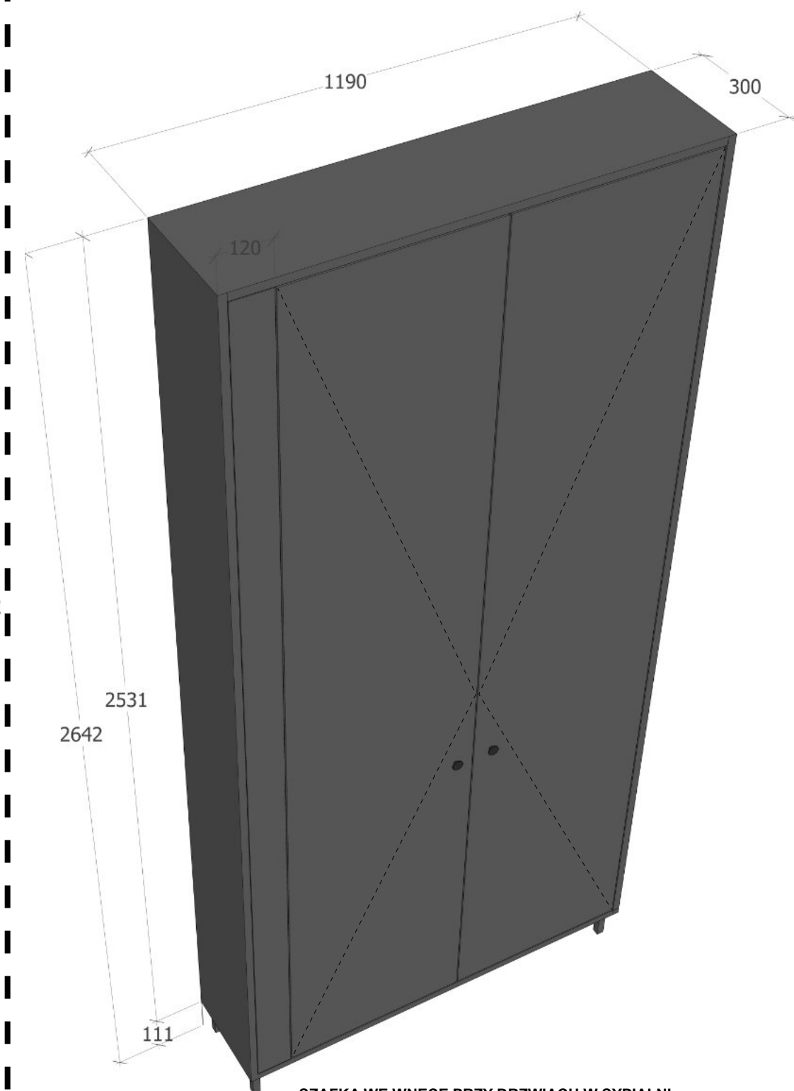
SZAFKA WE WNĘCE PRZY DRZWIACH W SYPIALNI
