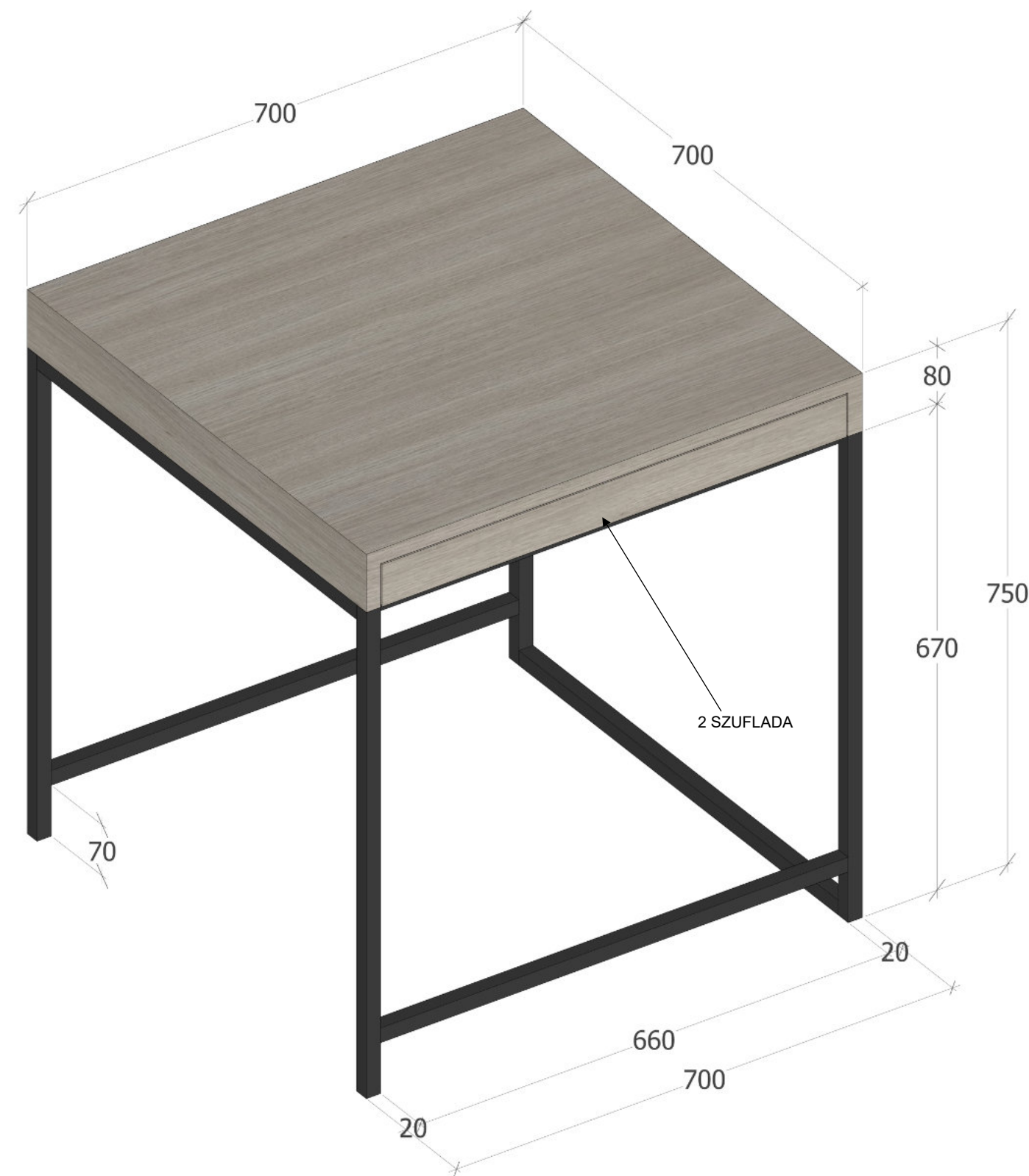
ELEMENT W9a - WIDOK 3D Z GÓRY
