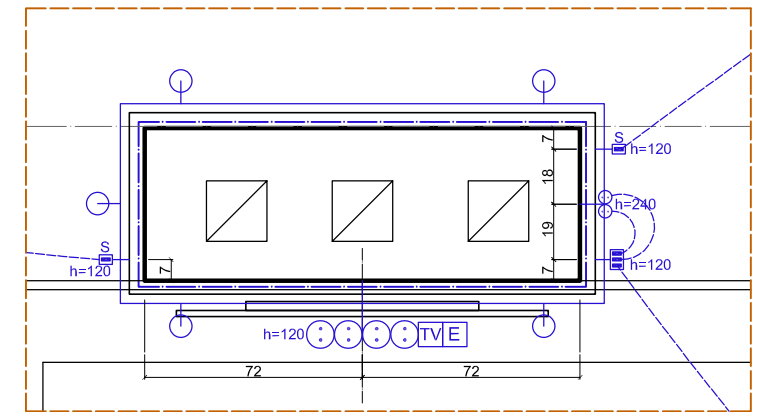
DETAL 1
